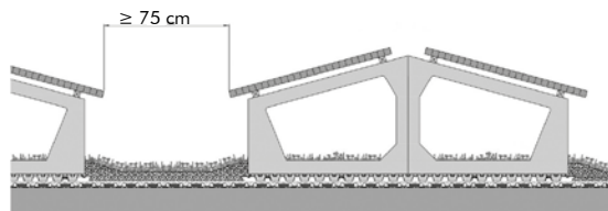
Solaraufständerung „Sattel“
