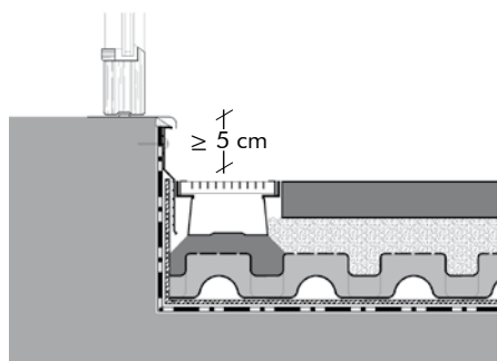
Tür Austritt auf Dächern. Als bewährte „Sonderlösung“ gemäß den Flachdachrichtlinien.
