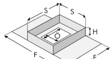
H = Höhe S = Schacht-Außenmaß F = Flansch Ö = Öffnungsmaß
