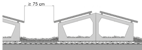
Solaraufständerung „Sattel“
