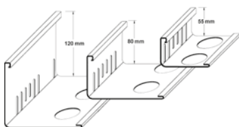
Stoßverbinder
