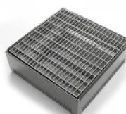
Kontrollschacht KS 6/30-GR und KS 10/30-GR mit herausnehmbarem feuerverzinktem Gitterrost
