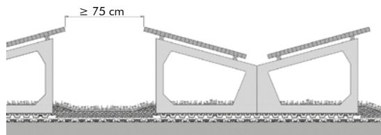
Solaraufständerung „Schmetterling“
