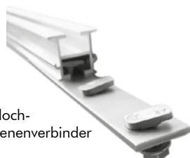
Solar-Montageprofil SMP 38/33
