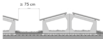
Solaraufständerung „Sattel“
