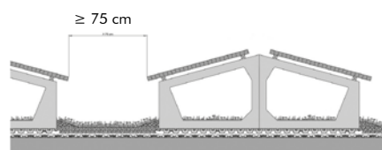
Solaraufständerung „Sattel“
