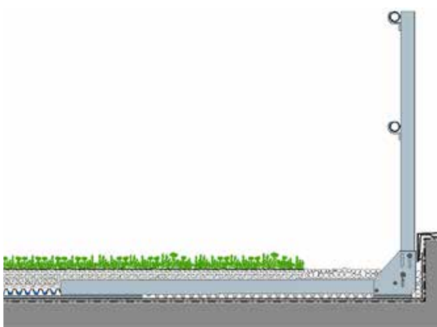
Fallnet® ASG Pfostenmodul Geländerholm
