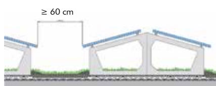
Solaraufständera „Sattel“
