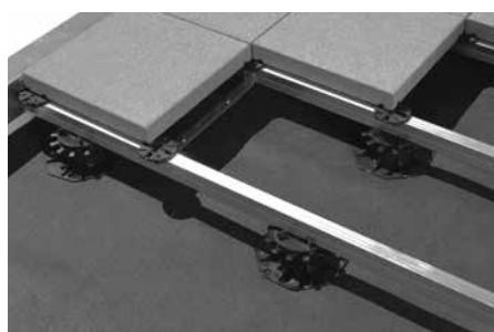
Verlegebeispiel
