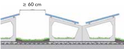
Solaraufständera „Schmetterling“
