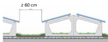
Solaraufständerung „Schmetterling“
