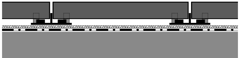
Elastoring - Plattenlager Höhe ca. 5, 10, 15 oder 20 mm
