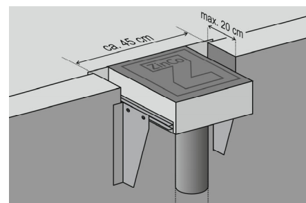
Ansicht geschlossen
